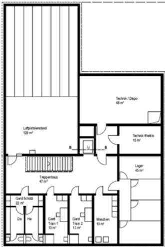
Grundriss UG
